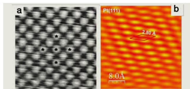
Fig. 6. Due esempi di immagini STM su superfici metalliche: (a) immagine STM ( 2,5 \times 2,5 \text{ nm} ; I = 1 \text{ nA} , V_{bias} = 1,1 \text{ V} ) di un campione di NiO dove sono visibili solo gli atomi di Ni (da Rif [12]); (b) Immagine STM di una superficie pulita di Pt(111) ( 4 \text{ nm} \times 4 \text{ nm} , I = 49 \text{ pA} , V_{bias} = +48 \text{ mV} ) (da Rif [13])
