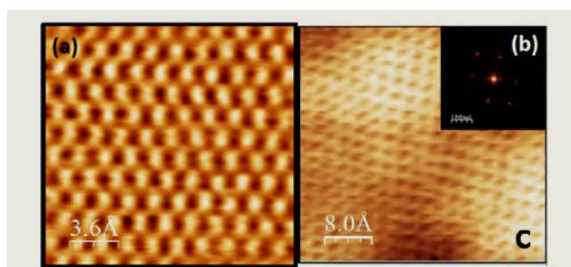
Fig. 10 (a) Immagine STM di un campione di grafite (18 × 18) Å, I = 1 \text{ nA} , V = 0,02 \text{ V} : è evidente la struttura esagonale centrata; (b) esagono nello spazio di Fourier ottenuto calcolando la FFT bidimensionale dell'immagine riportata in (c) che si riferisce ad una misura STM a corrente costante (40 × 40) Å, I = 1 \text{ nA} , V = 0,02 \text{ V} misurata su un campione di grafene cresciuto su una superficie di Ge(001) (da Rif. [15]); le misure STM sono state acquisite presso il NanoLab STM di Tor Vergata
