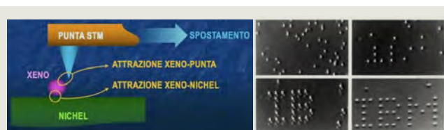
Fig. 14 Sequenza realizzata usando la punta del microscopio STM per spostare atomi di Xe su una superficie di Ni(110) (da Rif. [19]): fu la prima dimostrazione di nanomanipolazione a livello di singoli atomi; le lettere della scritta IBM hanno una dimensione di circa 50 Å
