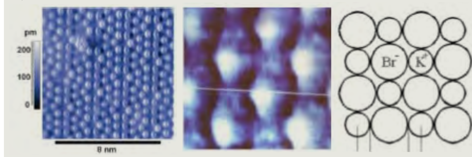
Fig. 19 In alto: immagini STM e AFM a confronto ottenute su grafite (parzialmente riprodotta dal Rif. 23); in basso: risoluzione atomica su Silicio (111) ricostruito (parzialmente riprodotta dal Rif. 24) e su un cristallo di KBr con vicino il modello per l'identificazione dei singoli atomi di Br e K del cristallo (parzialmente riprodotta dal Rif. 25)
