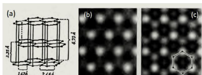
Fig. 8 (a) Struttura cristallografica di un campione di grafite: (b) e (c) sono due immagini a corrente costante misurate con diversi valori di tensione di bias (da Rif [14]); in un caso si vedono solo 3 dei 6 atomi della struttura esagonale di superficie, mentre nel secondo caso si vedono tutti e 6 gli atomi ma la loro intensità è modulata
